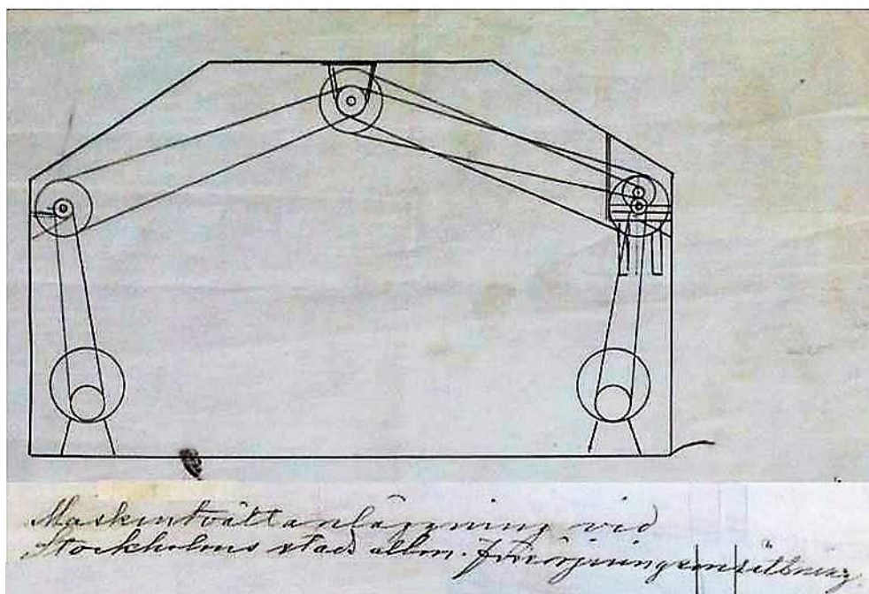
Fig. 18 39) Remdrift av "Maskintvätt- anläggning vid Stockholms stads allm. försörjnings- inrättning"
