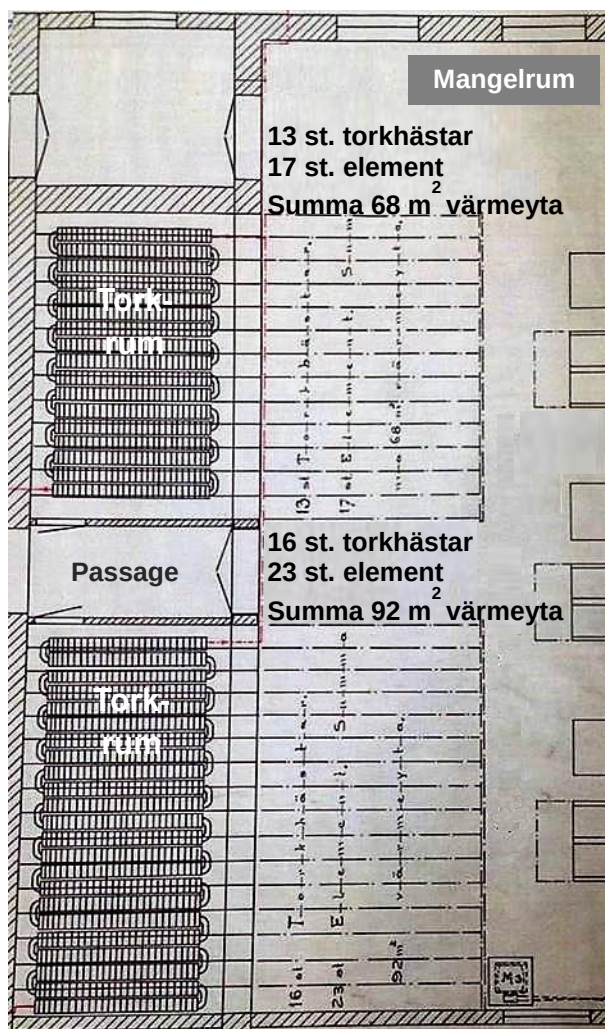
Fig. 14 34) Torkanordningen i Torkuset
