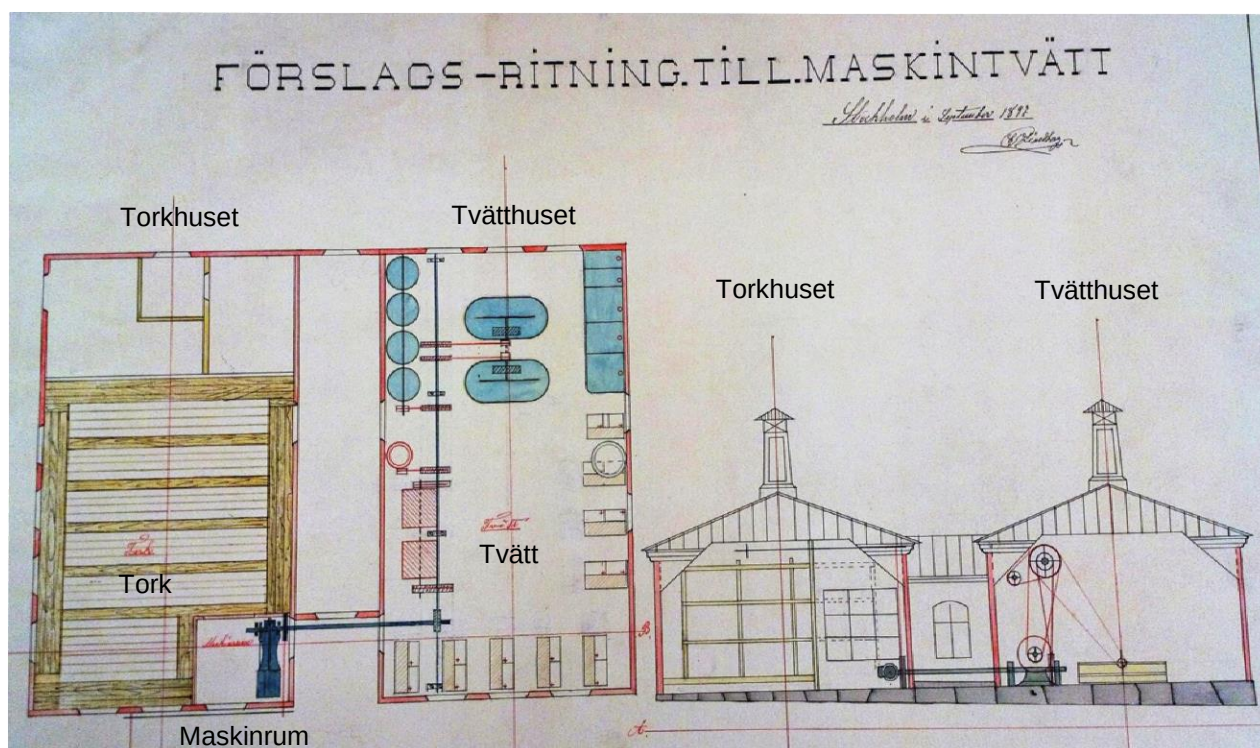
Fig. 11 27) Inredningen i Tvätthuset och Torkhuset
