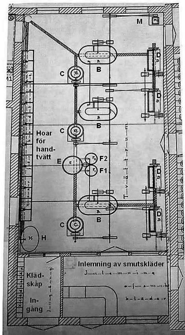
Fig. 15 34) Maskinuppställningen i Tvätthuset
